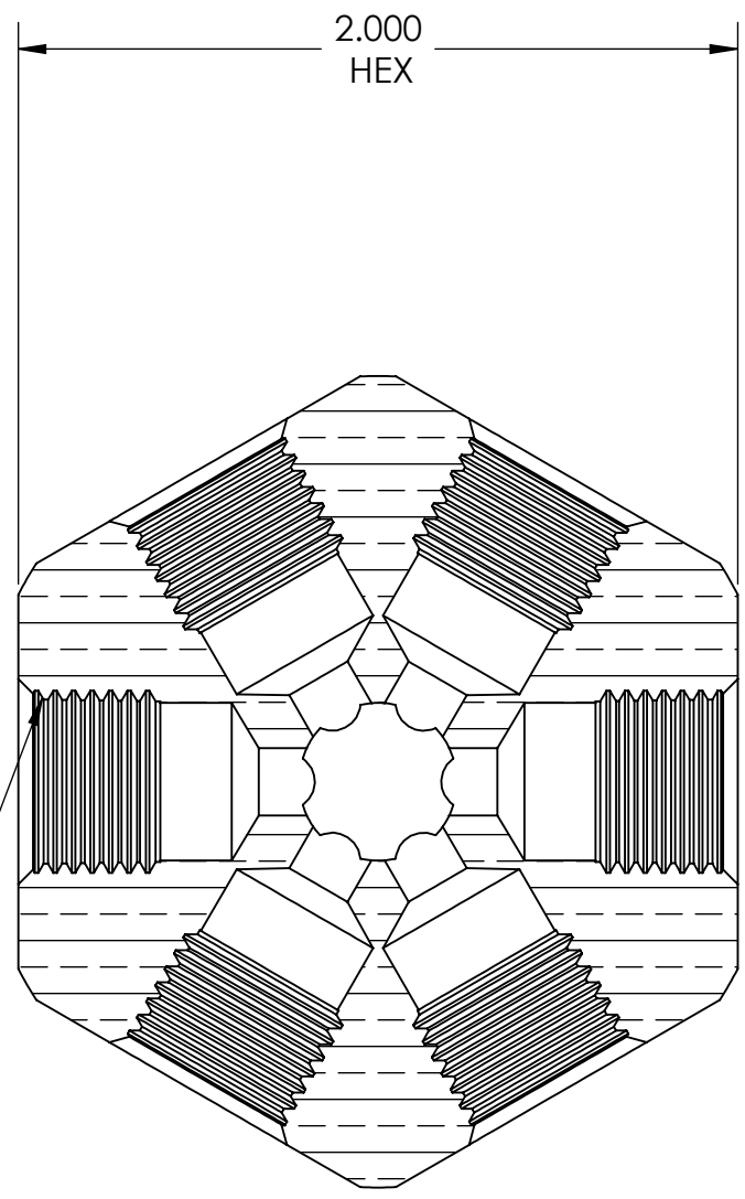
SECTION A-A SCALE 1.7 : 1
